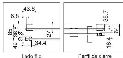
Dibujo técnico TN102 Frente de Ducha
