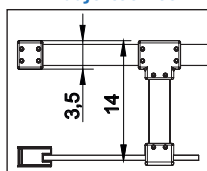
Detalle fijación barra a pared
