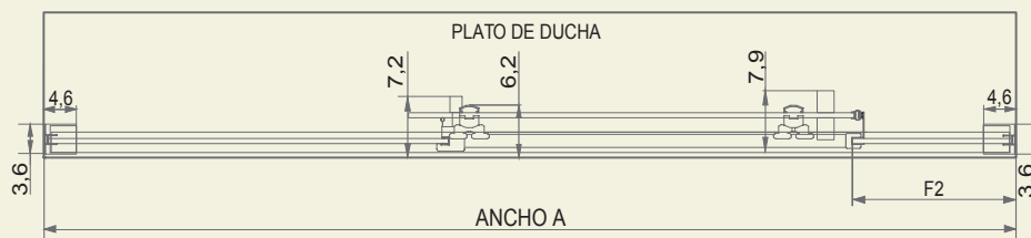
Dibujo técnico SU107
