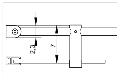
Detalle fijación barra a pared
