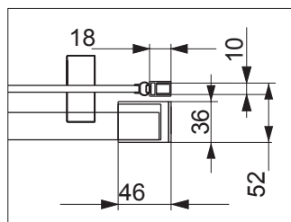
Perfil de cierre
