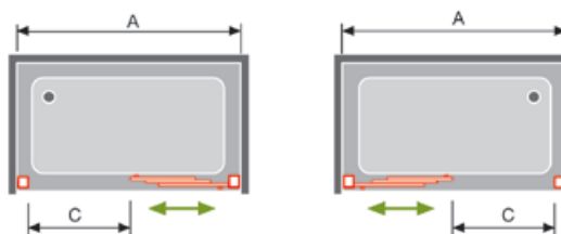
Dibujo técnico BN101 Frente de Ducha
