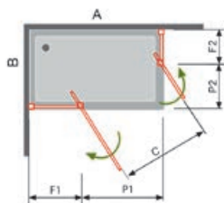
Dibujo técnico
