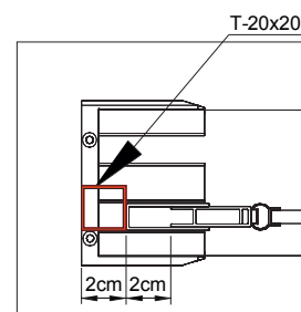
Detalle del tubo para incrementar medida
