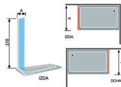
Dibujo técnico TN102
