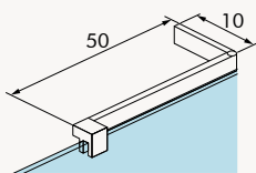
Barra paralela de fijación cromo Chrome support parallel bar Barre de fixation parallèle chrome
