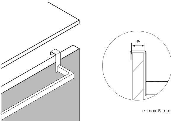
Toallero lateral
