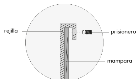
Rejilla esquinera
