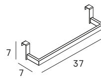
Toallero lateral
